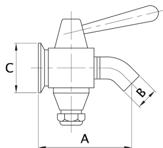
วาล์วสำหรับตรวจสอบคุณภาพ, 304 AND 316L, TYPE A
