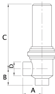
วาล์วกันกลับสแตนเลสหรือ เช็ควาล์วสแตนเลส , 316L
